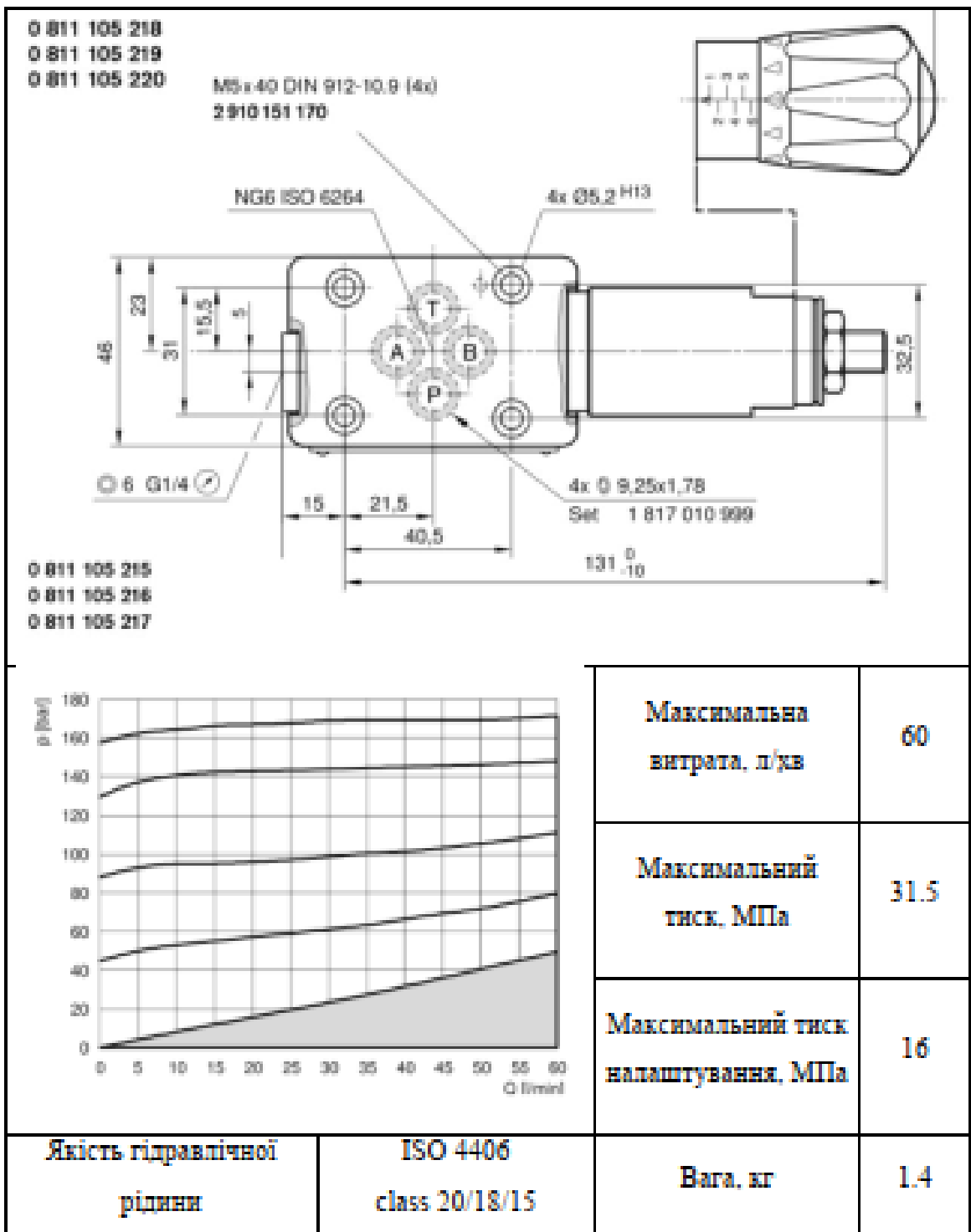
Рис. 4.8. Клапан тиску KT2 Bosch Rexroth DB6DPBW7-1X/160V.
