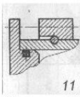
Кріплення кришок 11
