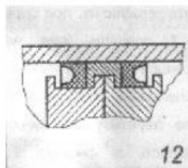
Ущільнення поршня 12
