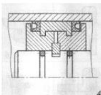
Кріплення поршня до штока 3
